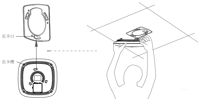
图3-5 安装AP到安装架示意图
